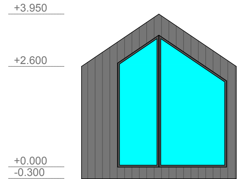
FASĀDE ASĪS 1-2
